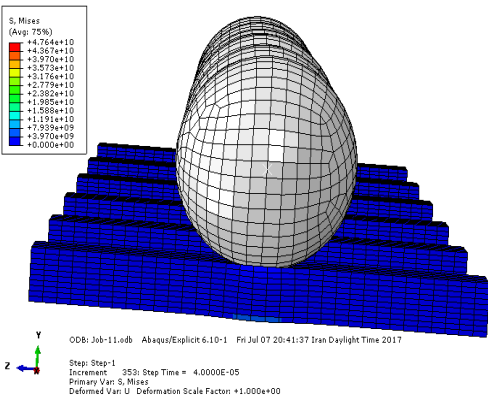
شکل ۲- نمای از شش تیر تحت بار ضربه توسط گلوله و المان‌بندی شده منبع: نرم افزار آباکوس
