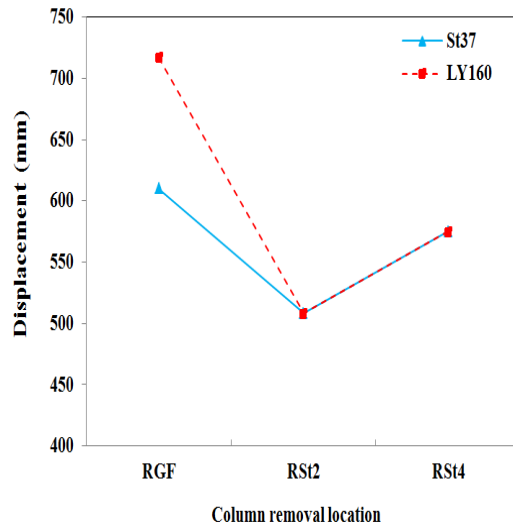
شکل ۱۴- مقایسه بیشینه جابجایی محل حذف ستون در قاب ۶ طبقه با بررسی نوع فولاد در اتصال RBS
