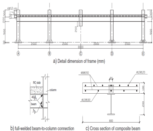
شکل ۳- جزئیات و ابعاد قاب
