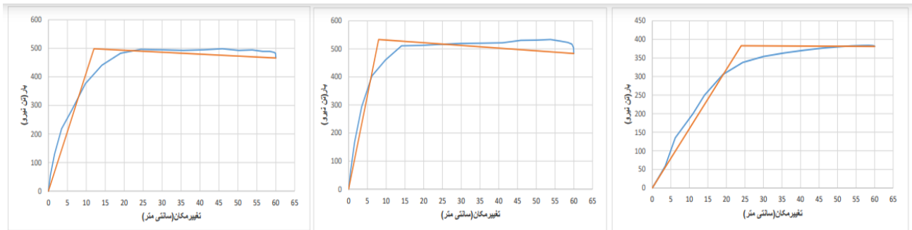
نمودار منحنی بار-تغییر مکان قاب خمشی ویژه ۸ طبقه دارای دیوار برشی با بازشوهای مستطیلی
