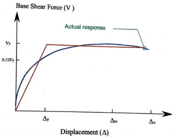
شکل ۸- روش دوخطی کردن نمودار پوش آور پریستلی و پائولی [۱۷]
