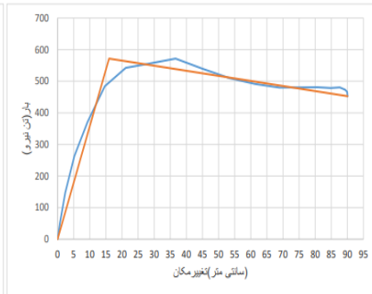
نمودار منحنی بار-تغییر مکان قاب خمشی ویژه ۱۲ طبقه دارای دیوار برشی
