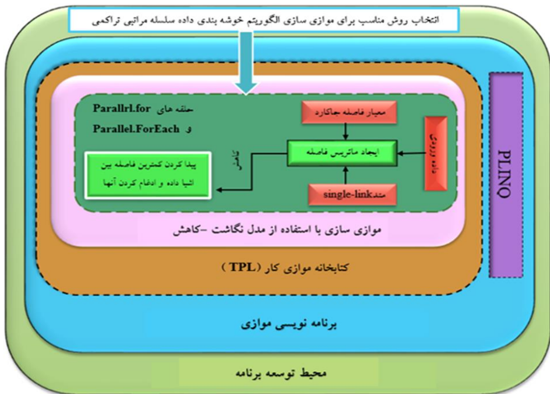
شکل (۴): مراحل توسعه الگوریتم ترتیبی خوشه‌بندی سلسله‌مراتبی تراکمی به صورت موازی
