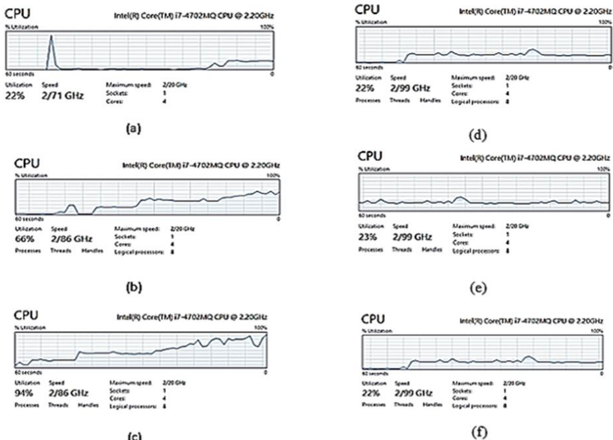
شکل (۱۲): وضعیت پردازنده سیستم در روش موازی (a,b,c) و روش ترتیبی (d,e,f) Figure (12): The processor status in the parallel method (a, b, c) and the sequential method (d, e, f)
