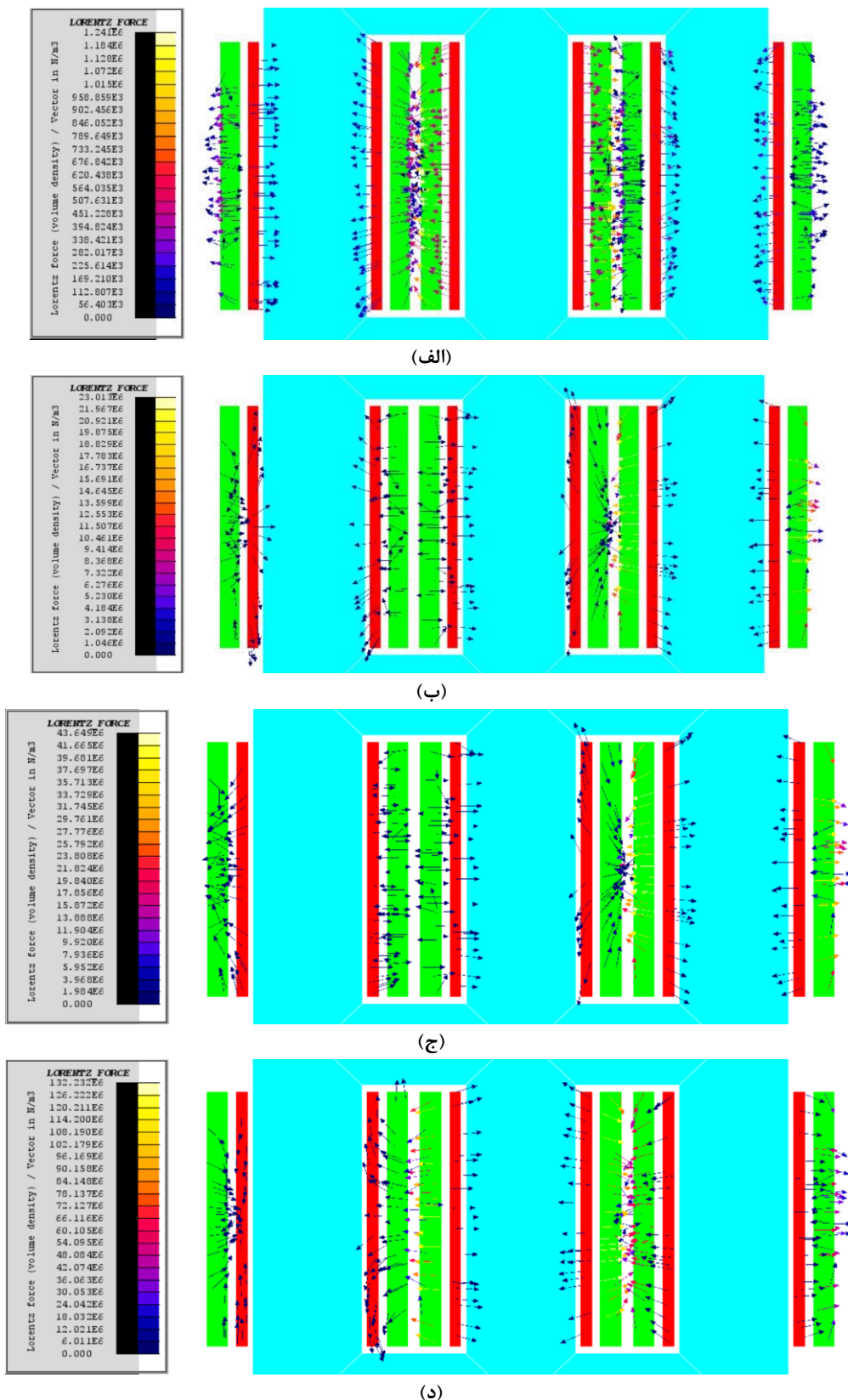
شکل (۸): توزیع بردارهای چگالی نیروهای لورنتس در حالات زمانی مختلف: الف) قبل از خطا ( t=0.034 s)، ب) بعد از قطع فاز اول ( t=0.13 s)، ج) بعد از قطع فاز دوم ( t=0.15 s)، د) بعد از قطع فاز سوم ( t=0.29 s) Fig. (8): The distribution of the Lorentz forces density at the different states: a) Before fault, b) After first phase cutting off, c) After second phase cutting off, d) After third phase cutting off
