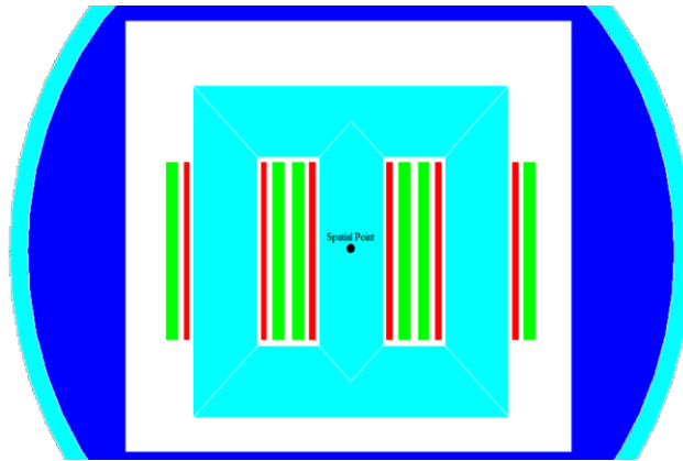
شکل (۲): مدل اجزای محدود دو بعدی ترانسفورماتور توزیع Fig. (2): The 2D finite element model of distribution transformer
