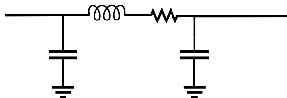
شکل (۳): مدل \pi خط انتقال متوسط Fig. (3): The \pi model of medium voltage transmission network
