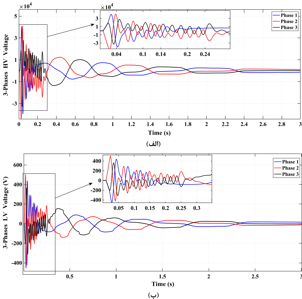
شکل (۵): شکل موج‌های ولتاژ: الف) اولیه، ب) ثانویه
