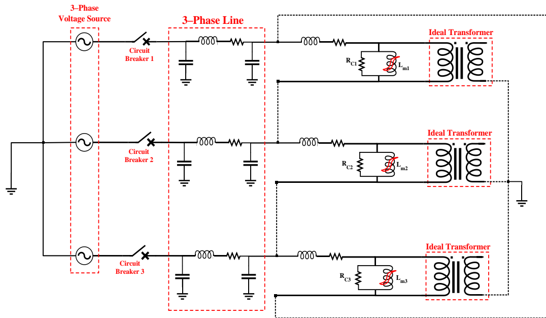
شکل (۴): مدار معادل خط و ترانسفورماتور سه‌فاز برای بررسی پدیده فرورزونانس Fig. (4): The equivalent circuit model of 3-phase power system and transformer for ferroresonance study
