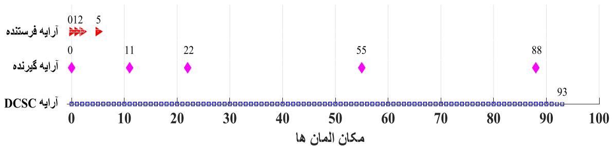
شکل (۳): مثالی از یک رادار MIMO با ۴ المان فرستنده، ۵ المان گیرنده و فاصله بین المانی ۱۱ Figure (3): An example of MIMO radar with 4 elements receiver, 5 elements transmitter and inter-element space 11
