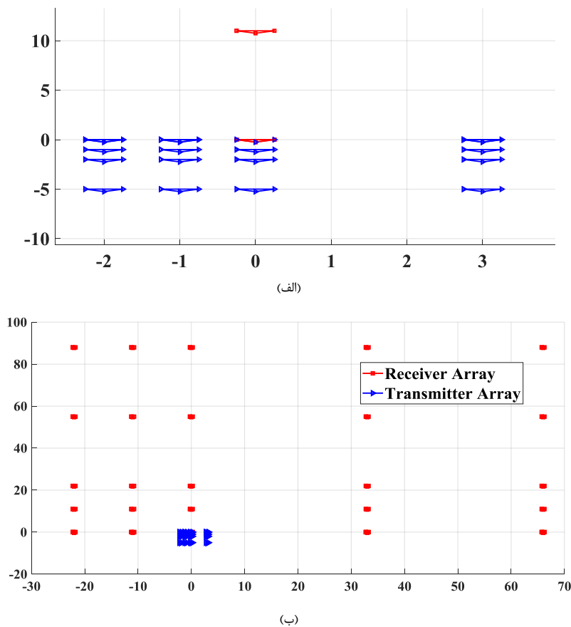
شکل (۷): چینش آرایه فیزیکی فرستنده و گیرنده پس از شیفت (الف) شکل بزرگنمایی شده جهت مشاهده بهتر آرایه فرستنده (ب) شکل کلی فرستنده و گیرنده همزمان
