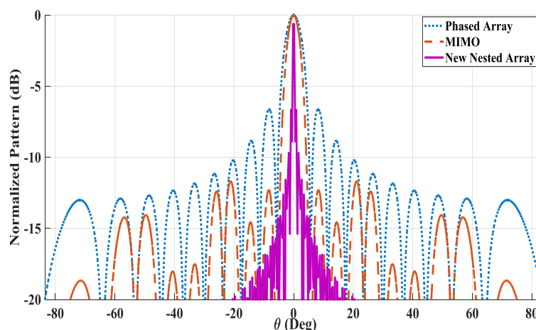
شکل (۴): پترن چینش‌های مختلف آرایه Figure (4): Pattern of different array configuration
