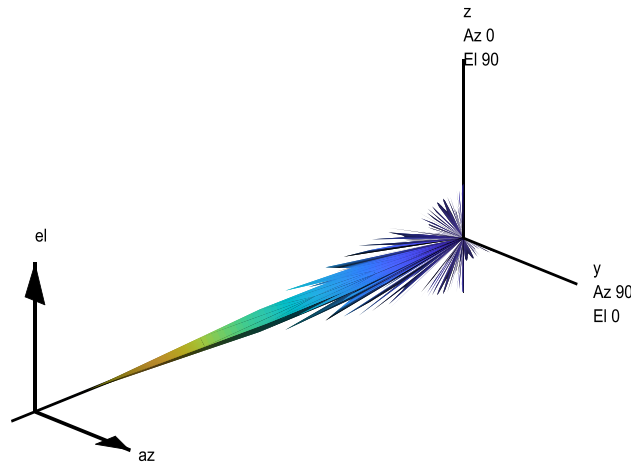
شکل (۹): الگوی تشعشعی سه‌بعدی ناشی از چینش تودرتوی دوبعدی با ۱۶ المان فرستنده و ۲۵ المان گیرنده
