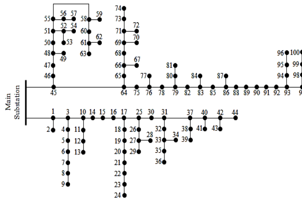
شکل (۴): دیاگرام تک خطی سیستم توزیع ۱۰۱ شینه شهرک صنعتی خوی، ایران [۲۴] Figure (4): The single line diagram of actual 101 bus distribution system in Khoys, Iran [24]
