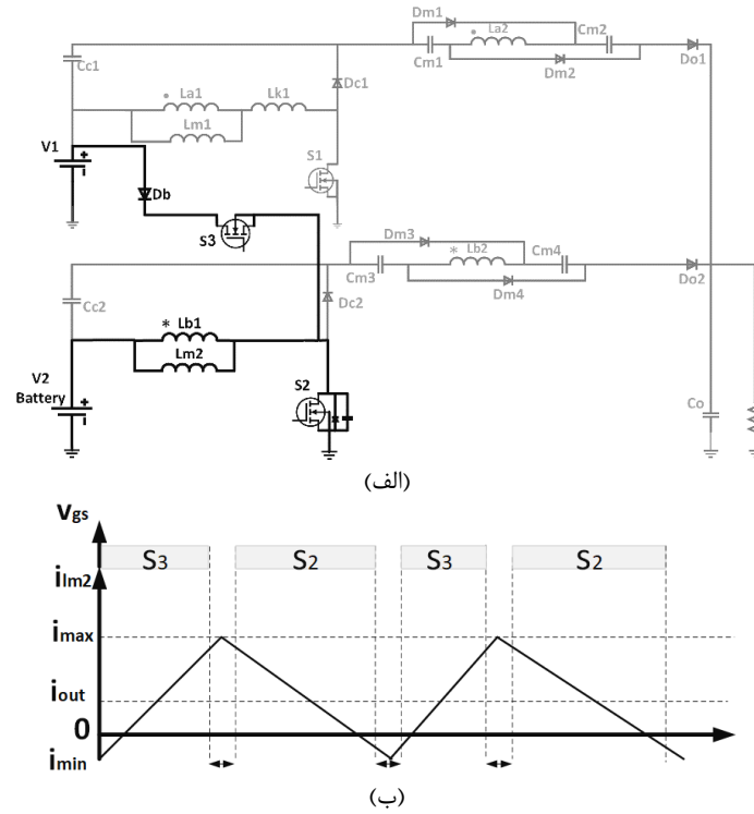
شکل (۶): اجزای مبدل که به شارژ سیستم ذخیره انرژی کمک می‌کند
