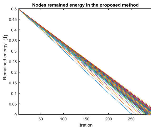
شکل (۳): انرژی باقیمانده گره‌های حسگر
