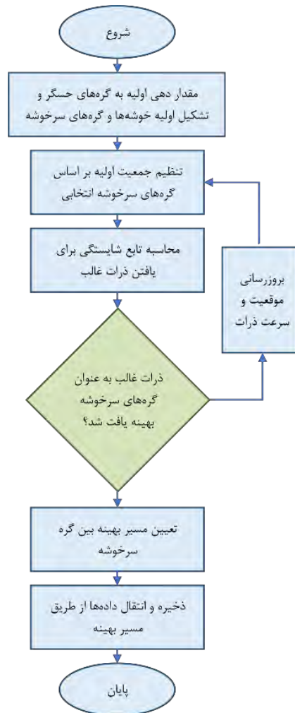
شکل (۲): فلوچارت روش پیشنهادی
