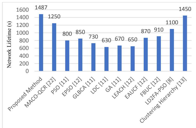
شکل (۱۰): مقایسه روش پیشنهادی و سایر روش‌ها از نظر طول عمر شبکه
