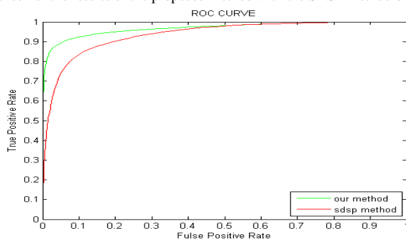
شکل (۶): مقایسه منحنی ROC روش پیشنهادی با روش SDSP بر روی تصاویر حاوی بافت در پایگاه داده MSRA10K Figure (6): Comparison of ROC curve of proposed method with SDSP method on images containing texture in MSRA10K database
