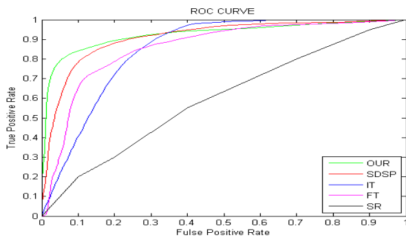
شکل (۴): مقایسه منحنی ROC مدلها بر روی پایگاه داده MSRA10K Figure (4): Comparison of ROC curves of models on MSRA10K database
