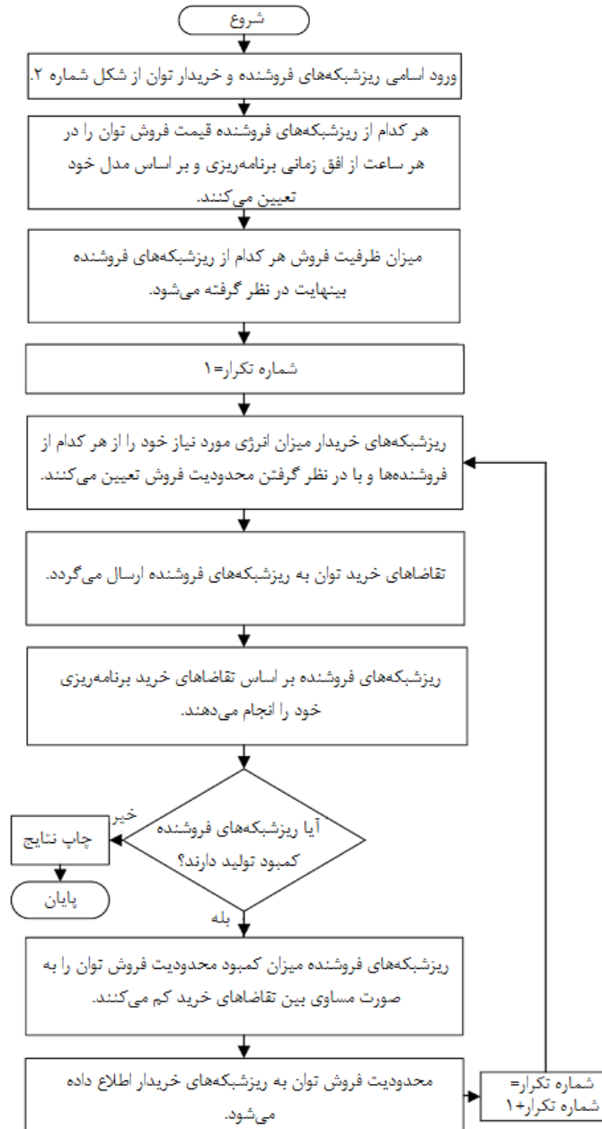
شکل (۳): روندنمای الگوریتم غیرمتمرکز پیشنهادی Figure (3): Flowchart of proposed decentralized algorithm
