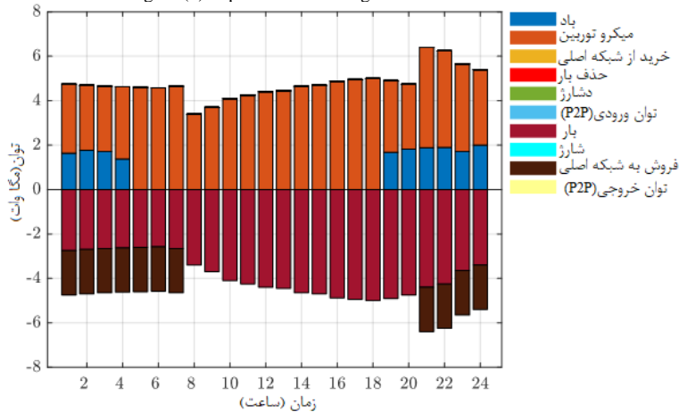
شکل (۸): بهره برداری از ریزشبهه شماره چهارده در سناریوی اول
