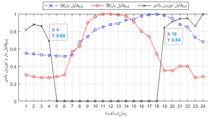
شکل (۵): میزان بار مصرفی شبکه و تولید توربین های بادی [۱]
