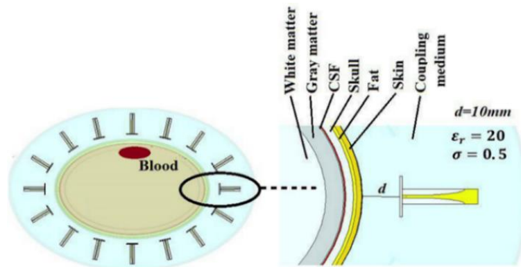
شکل (۱): طراحی و نحوه چیدمان آنتن‌ها در تصویربرداری میکروویو از مغز Figure (1): The proposed microwave imaging setup and design of the antenna.
