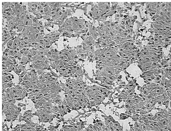
شکل میکروسکوپی فتوکروموسیتوم رنگ آمیزی شده با هماتوکسیلین و اوژین
