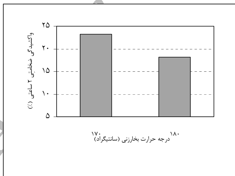
شکل شماره ۴- اثر درجه حرارت بخارزنی بر واکشیدگی ضخامتی پس از ۲ ساعت
