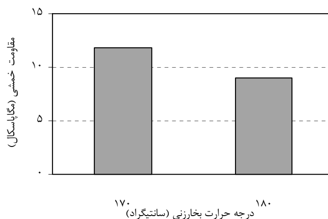
کل شماره ۱۱- اثر درجه حرارت بخارزنی بر مقاومت خمشی
