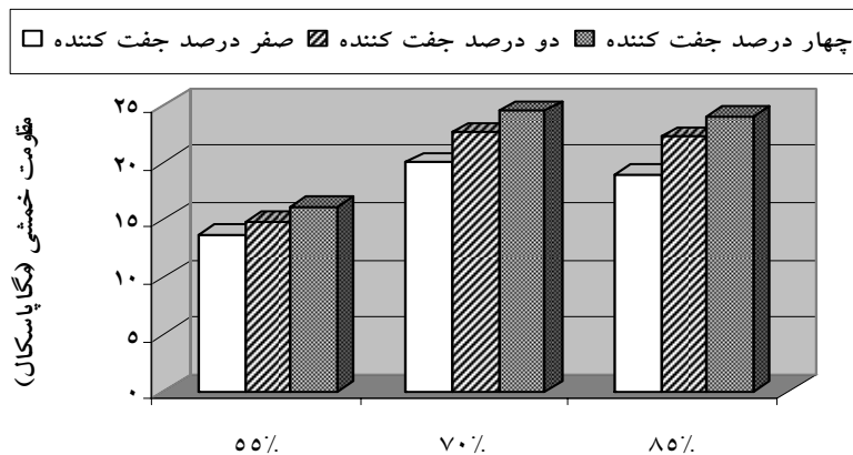
شکل ۳ - اثر متقابل میان درصد الیاف کارتن کهنه و درصد عامل جفت‌کننده بر مقاومت خمشی در کامپوزیت
