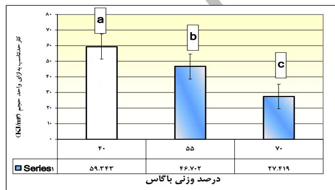
شکل ۷- اثر مستقل مقدار الیاف بر کار حدتناسب خمشی تخته‌های آزمون
