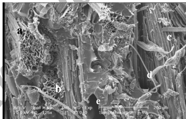
شکل ۱۱- تصویر SEM از تیمار ۴۰ درصد الیاف و ۴ درصد سازگارکننده
