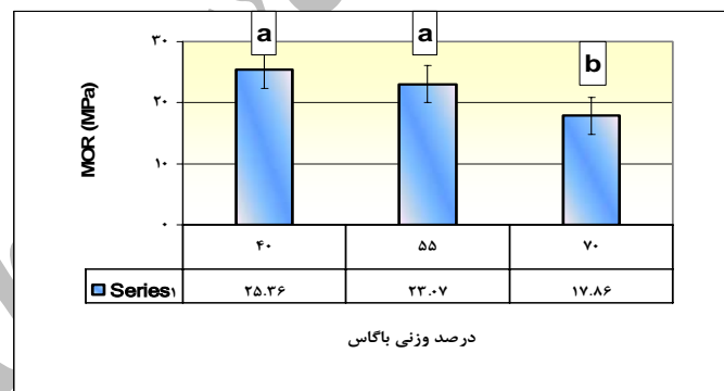
شکل ۱- اثر مستقل مقدار الیاف بر مدول گسیختگی تخته های آزمونی
