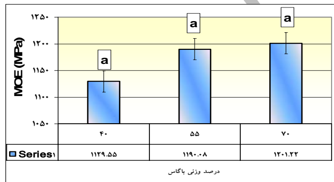
شکل ۴- اثر مستقل مقدار لیاف بر مدول الاستیسیته تخته‌های آزمون
