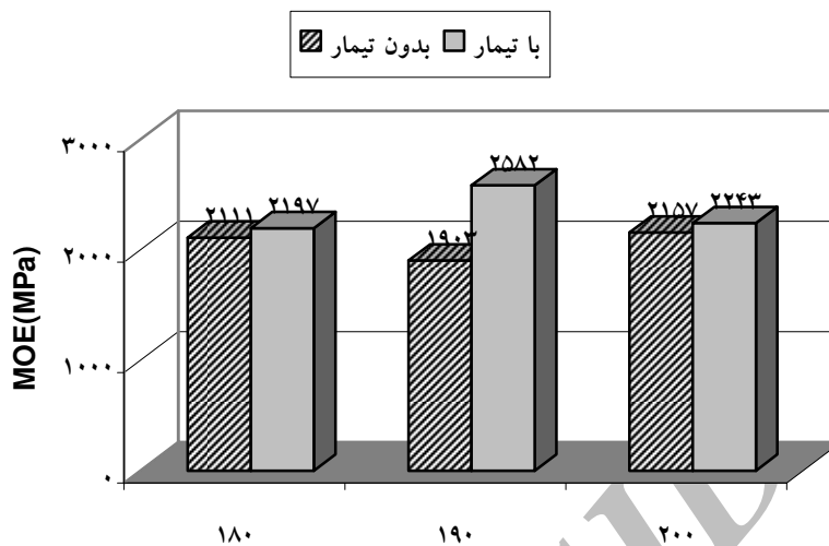
شکل 2 - اثر متقابل میان تیمار اصلاحی انیدرید مالیک و دمای پرس بر مدول خمشی تخته فیبر با دانسیته متوسط
