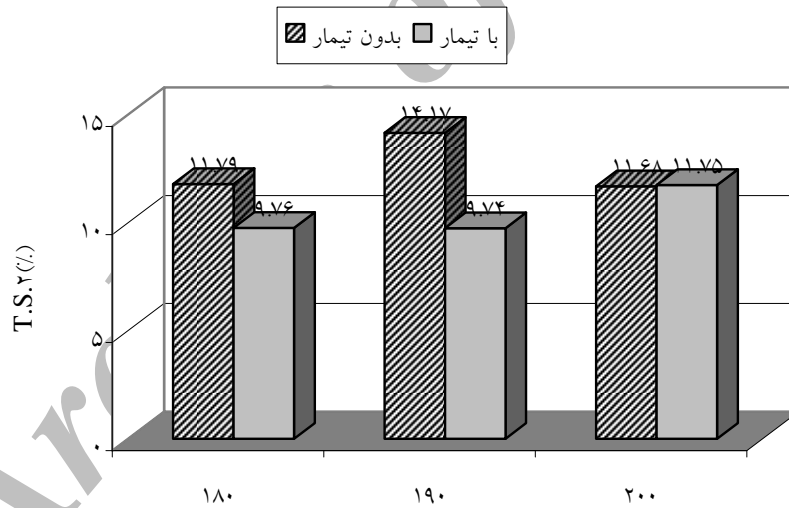
شکل 4 - اثر متقابل میان تیمار اصلاحی انیدرید مالییک و دمای پرس بر واکنشیدگی ضخامت پس از 2 ساعت غوطه وری در آب در تخته فیبر با دانسیته متوسط
