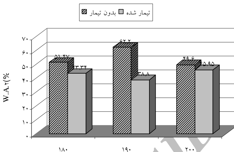
شکل 6 - اثر متقابل میان تیمار اصلاحی انیدرید مالیک و دمای پرس بر جذب آب پس از 2 ساعت غوطه وری در آب در تخته فیبر با دانسیته متوسط
