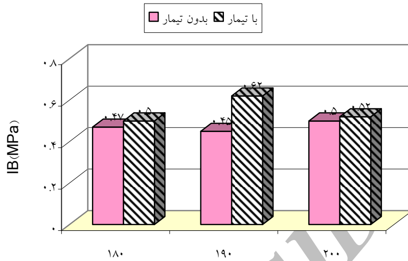
شکل 3 - اثر متقابل میان تیمار اصلاحی انیدرید مالییک و دمای پرس بر چسبندگی داخلی تخته فیبر با دانسیته متوسط
