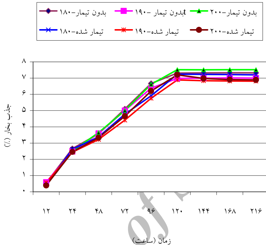
شکل 8 - اثر تیمارهای اصلاحی انیدرید مالیک و دمای پرس بر جذب رطوبت طولانی مدت در تخته فیبر با دانسیته متوسط
