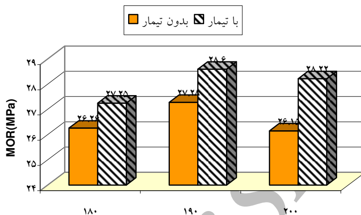
شکل 1 - اثر متقابل میان تیمار اصلاحی انیدرید مالیک و دمای پرس بر مقاومت خمشی تخته فیبر با دانسیته متوسط
