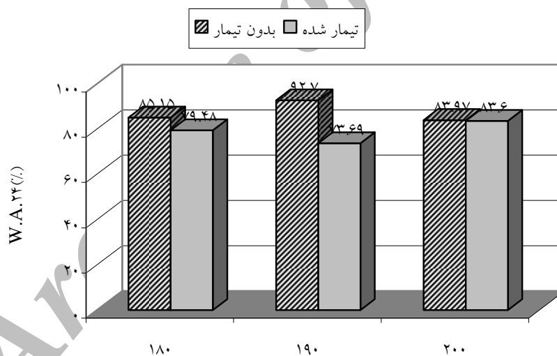
شکل 7 - اثر متقابل میان تیمار اصلاحی انیدرید مالیک و دمای پرس بر جذب آب پس از 24 ساعت غوطه وری در آب در تخته فیبر با دانسیته متوسط
