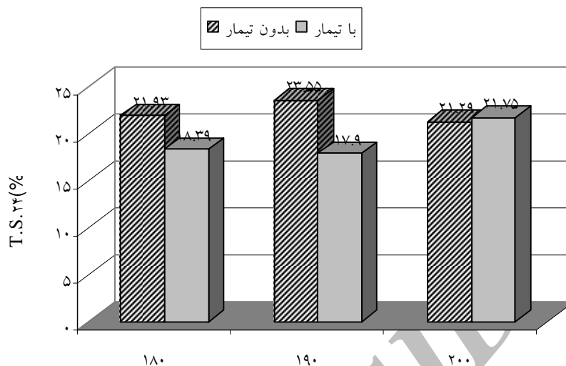
شکل 5 - اثر متقابل میان تیمار اصلاحی انیدرید مالیک و دمای پرس بر واكشیدگی ضخامت پس از 24 ساعت غوطه وری در آب در تخته فیبر با دانسیته متوسط
