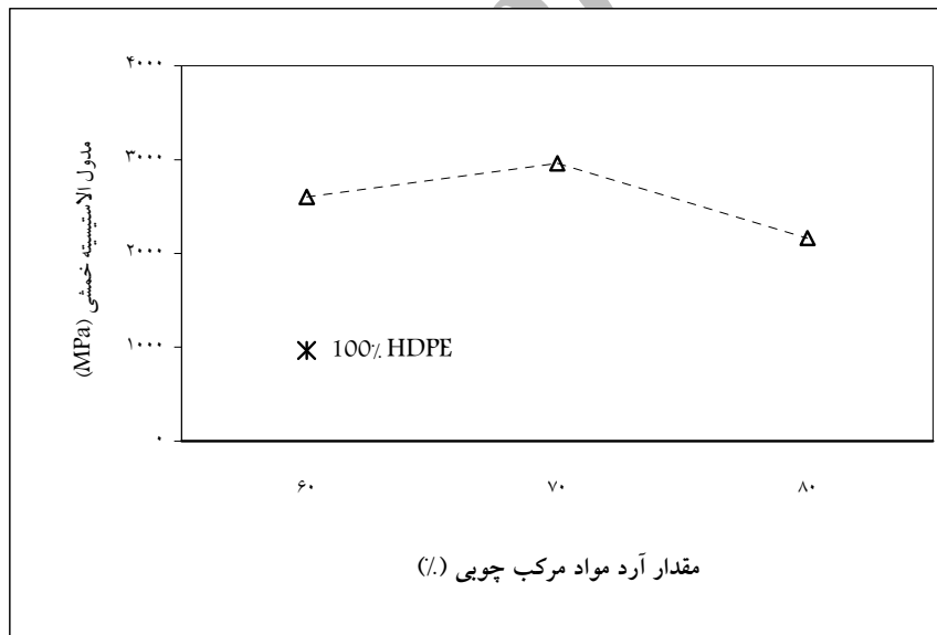
شکل 1- اثر مقدار مخلوط آرد تخته خرده چوب و تخته فیبر نیمه سنگین بر مدول الاستیسیته مواد مرکب چوب - پلاستیک
