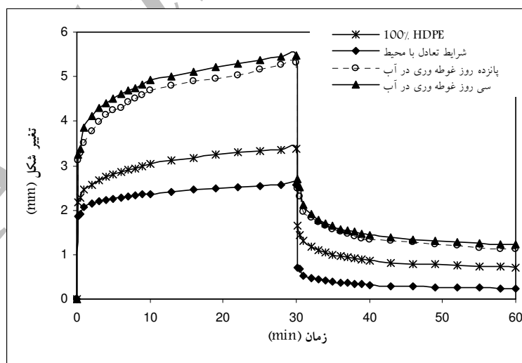
شکل 5- اثر زمان غوطه‌وری در آب بر رفتار خزش مواد مرکب چوب - پلاستیک (مقدار 60٪ مخلوط آرد تخته خرد چوب و تخته فیبر نیمه سنگین)
