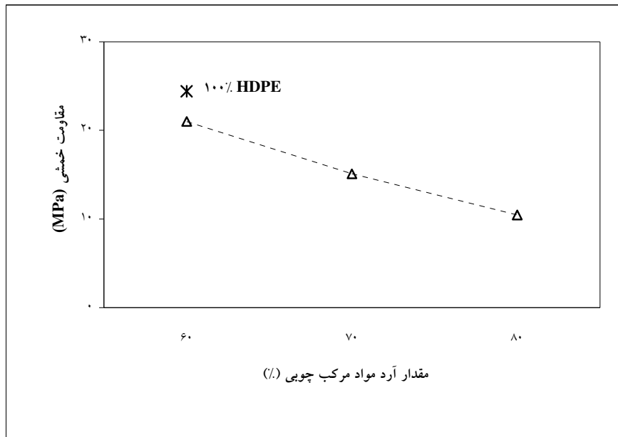
شکل 2- اثر مقدار مخلوط آرد تخته خرده چوب و تخته فیبر نیمه سنگین بر مقاومت خمشی مواد مرکب چوب - پلاستیک
