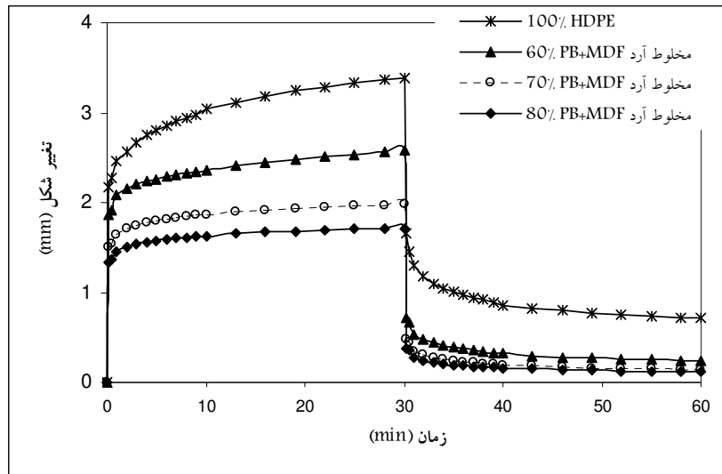
شکل 4- اثر مقدار مخلوط آرد تخته خرده چوب و تخته فیبر نیمه سنگین بر رفتار خزش مواد مرکب چوب - پلاستیک (شرایط تعادل با محیط)
