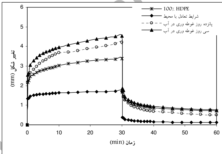
شکل 7: اثر زمان غوطه‌وری در آب بر رفتار خزش مواد مرکب چوب - پلاستیک (مقدار 80٪ مخلوط آرد تخته خرده چوب و تخته فیبر نیمه سنگین)
