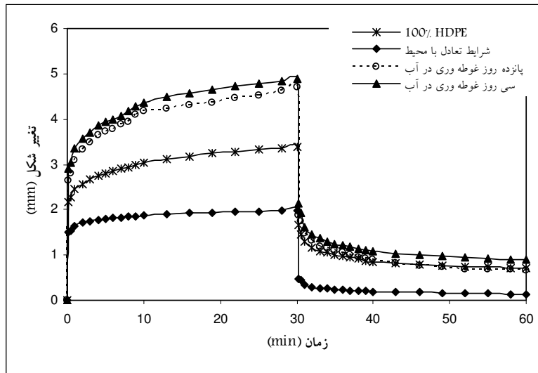
شکل 6: اثر زمان غوطه‌وری در آب بر رفتار خزش مواد مرکب چوب - پلاستیک (مقدار 70٪ مخلوط آرد تخته خرده چوب و تخته فیبر نیمه سنگین)
