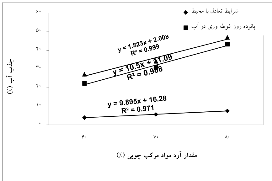
شکل 3- رابطه بین درصد جذب آب و مقدار مخلوط آرد تخته خرده چوب و تخته فیبر نیمه سنگین در مواد مرکب چوب - پلاستیک
