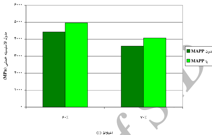
شکل 1- اثر عامل سازگارکننده بر روی مدول الاستیسیته خمشی
