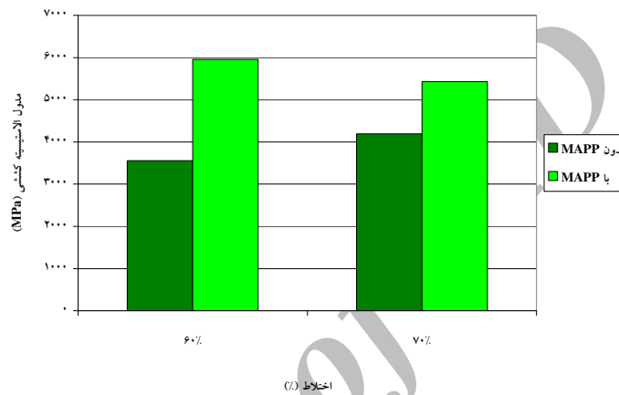
شکل 3- اثر عامل سازگارکننده بر روی مدول الاستیسیته کششی
