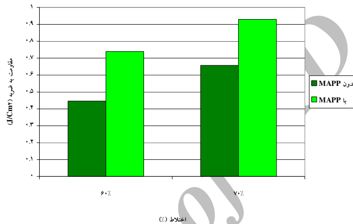
شکل 5- اثر عامل سازگارکننده بر روی مقاومت به ضربه
