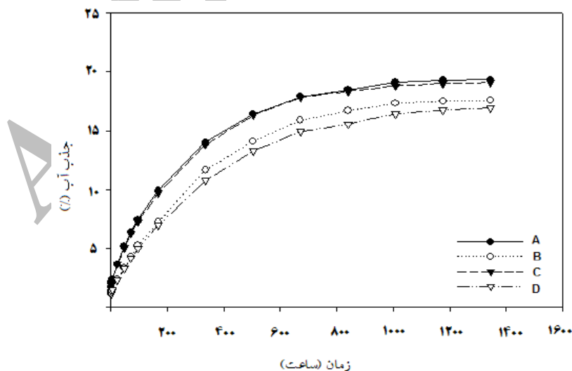
شکل 7- اثر عامل سازگارکننده بر میزان جذب آب ماده مرکب نی- پلی پروپیلن
