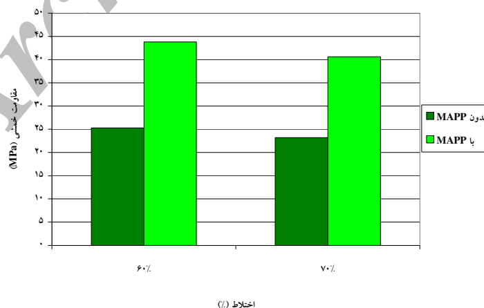
شکل 2- اثر عامل سازگارکننده بر روی مقاومت خمشی
