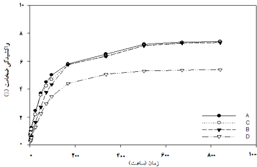
شکل 9- اثر عامل سازگارکننده بر میزان واکسیدگی ضخامت ماده مرکب نی- پلی پروپیلن در گوشه
