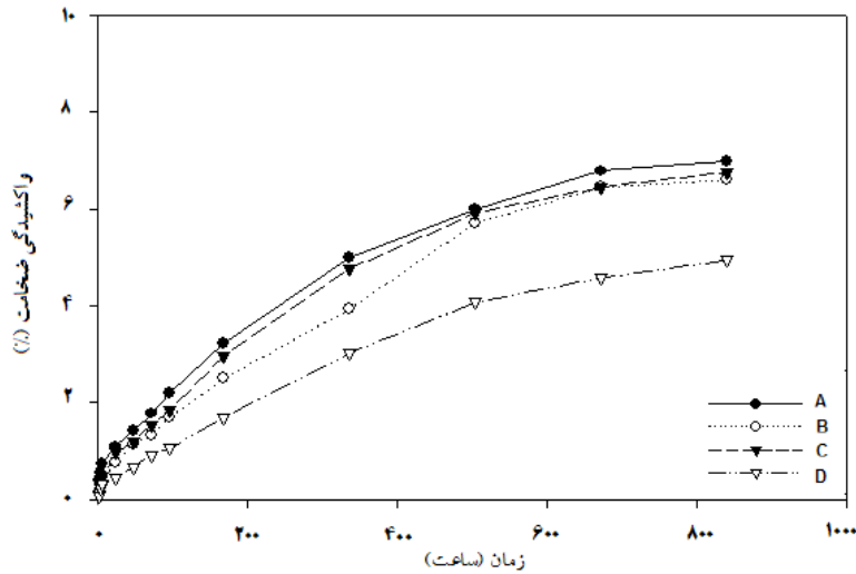
شکل 8- اثر عامل سازگارکننده بر میزان واکسیدگی ضخامت ماده مرکب نی- پلی پروپیلن در مرکز
