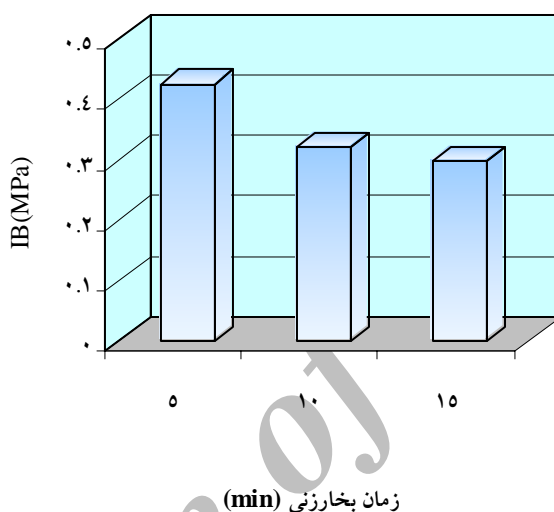
شکل ۳ - اثر زمان بخارزنی بر مقاومت چسبندگی داخلی
