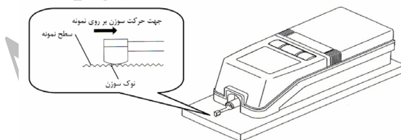
شکل ۱- طرح شماتیک از دستگاه Mitutoyo surftest SJ 201 و نوک اندازه‌گیری آن
