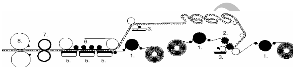
شکل ۱- شمایی از فرایند کنگره ای کردن کاغذ و ساخت ورق مقوای کنگره ای.
