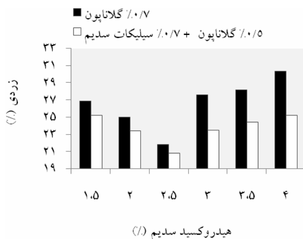
شکل ۱۴- تأثیر هیدروکسید سدیم بر زردی خمیرهای کاغذ CMP با پروکسید ۰/۳.
