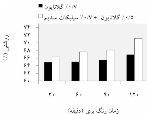
شکل ۱۹- تأثیر زمان رنگ بری بر روشنی خمیرهای کاغذ CMP با پروکسید ۰/۵٪ و هیدروکسید سدیم بهینه ۰/۲/۵٪
