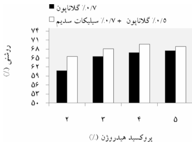
شکل ۱۶- تأثیر پروکسید هیدروژن بر روشنایی خمیرهای کاغذ CMP با مقدار بهینه هیدروکسید سدیم ۰.۲/۵.
