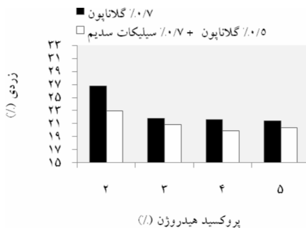
شکل ۱۷- تأثیر پروکسید هیدروژن بر زردی خمیرهای کاغذ CMP با مقدار بهینه هیدروکسید سدیم ۰.۲/۵.
