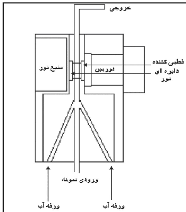
شکل ۱- پیکره‌بندی سلول جریان در تحلیل کیفیت الیاف (FQA)
