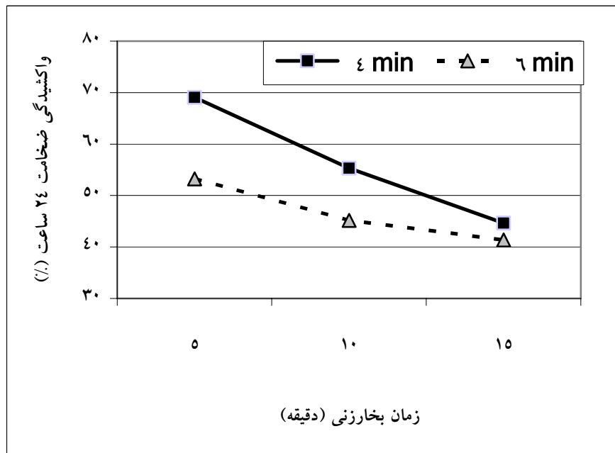
شکل ۷ - اثر متقابل زمان بخارزنی و زمان پرس بر واکسیدگی ضخامت ۲ و ۲۴ ساعت
