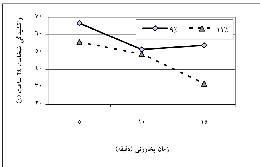
شکل ۶ - اثر متقابل زمان بخارزنی و مصرف چسب بر واکشیدگی ضخامت ۲ و ۲۴ ساعت
