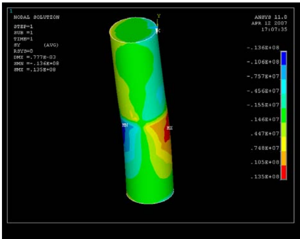
شکل ۴- تغییرات توزیع تنش در دوبل در بررسی مقاومت گشتاورخمش
