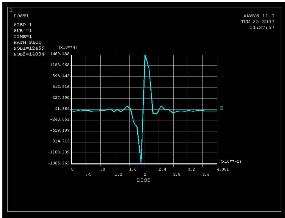
شکل ۵- تغییرات توزیع تنش در طول دوبل (بررسی مقاومت گشتاورخمش)
