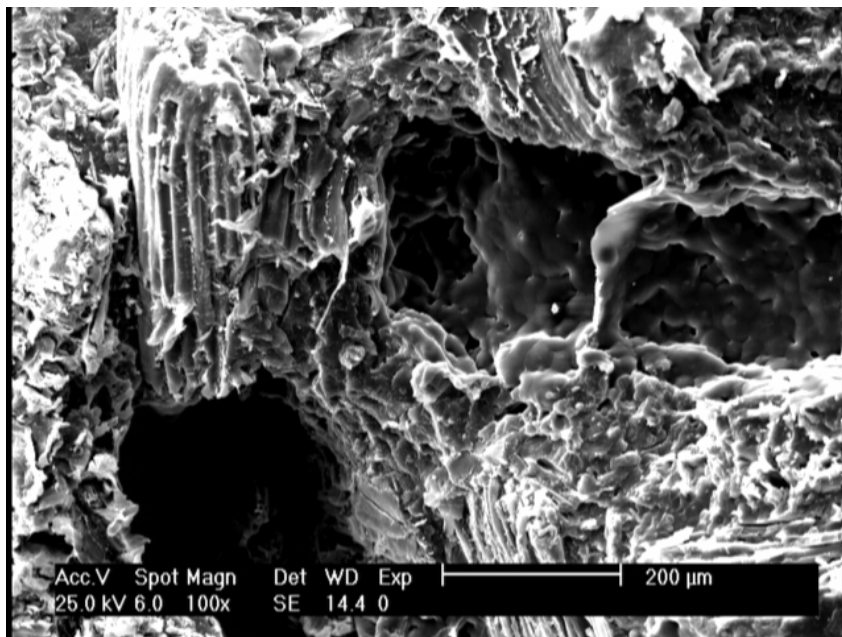
شکل ۷- سطح شکست نمونه کششی حاوی ۲ درصد نانو و گاه گندم
