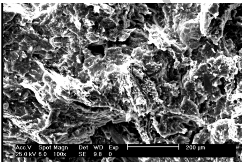
شکل ۸- سطح شکست کششی حاوی ۲ درصد نانو و گاه برنج
