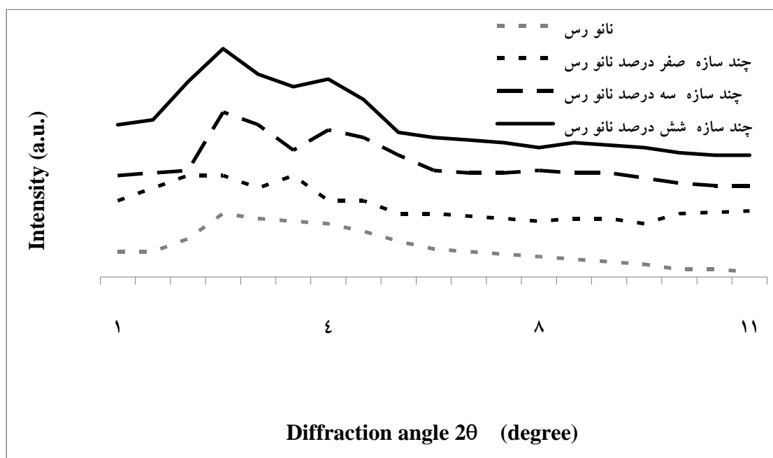
شکل ۱۰ - پراش اشعه ایکس در چندسازه ساخته شده در تیمارهای مختلف
