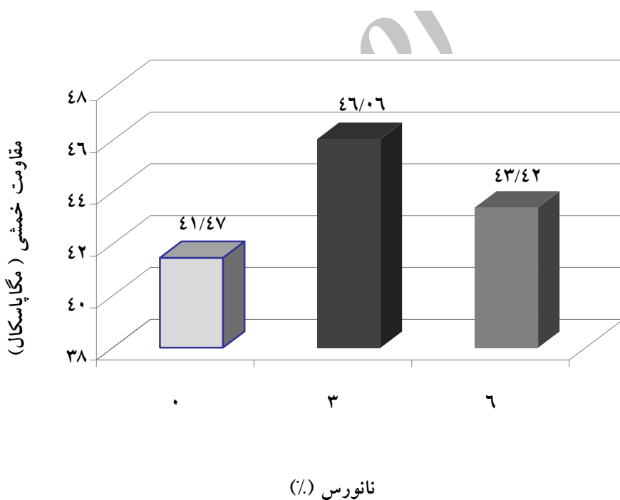
شکل ۶- اثر مستقل درصد نانورس بر مقاومت و مدول خمشی نانو چندسازه چوب پلاستیک
