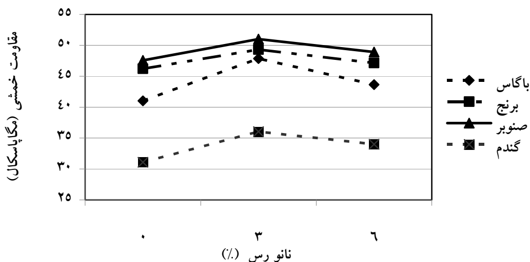
شکل ۷- اثر متقابل گونه چوبی و درصد نانورس بر مقاومت خمشى نانو چندسازه چوب پلاستیک
