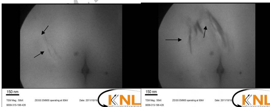
شکل ۱۲ - تصاویر میکروسکوپ الکترونی انتقالی نمونه‌های چندسازه چوب پلاستیک با بزرگنمایی ۱۵۰ نانومتر (تصویر سمت راست نمونه حاوی ۶ درصد نانورس / تصویر سمت چپ نمونه حاوی ۳ درصد نانورس)
