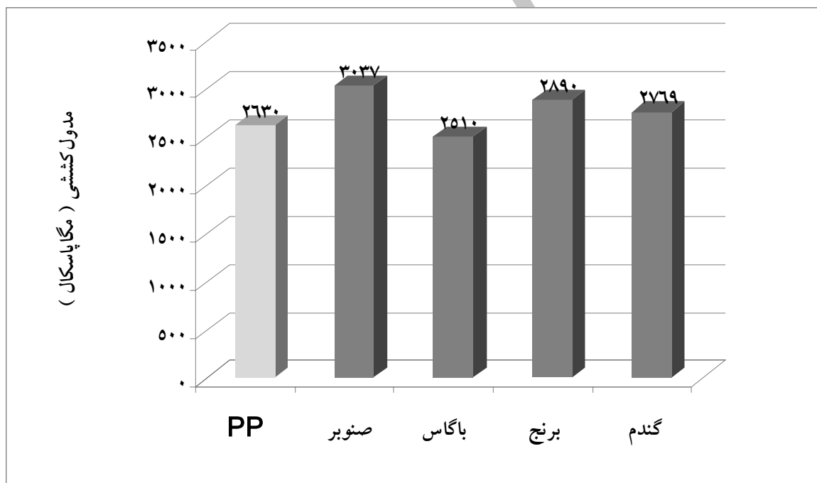
شکل ۲- اثر مستقل گونه چوبی بر مقاومت و مدول کششی نانو چندسازه چوب پلاستیک
