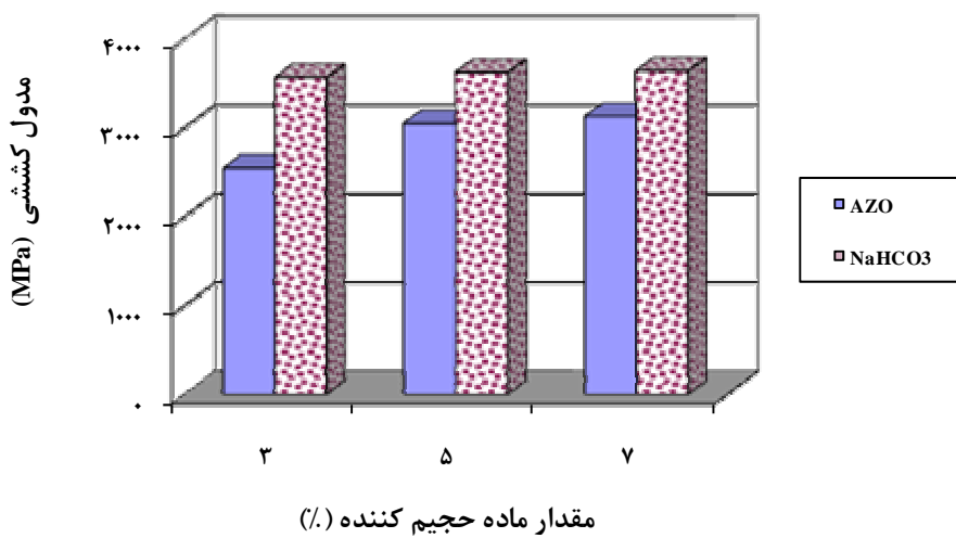
شکل ۵- تأثیر مقدار و نوع ماده حجیم کننده بر مدول کششی چندسازه الیاف OCC- پلی پروپیلن (مقدار الیاف OCC؛ ۲۰٪ و مقدار MAPP؛ ۳٪).
