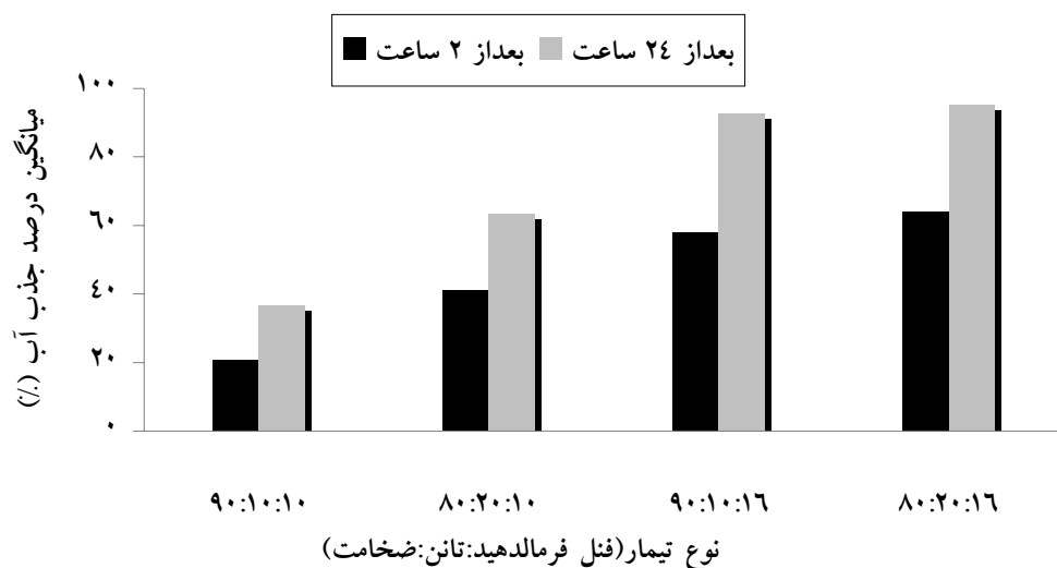
شکل ۵- نمودار میانگین درصد جذب آب
