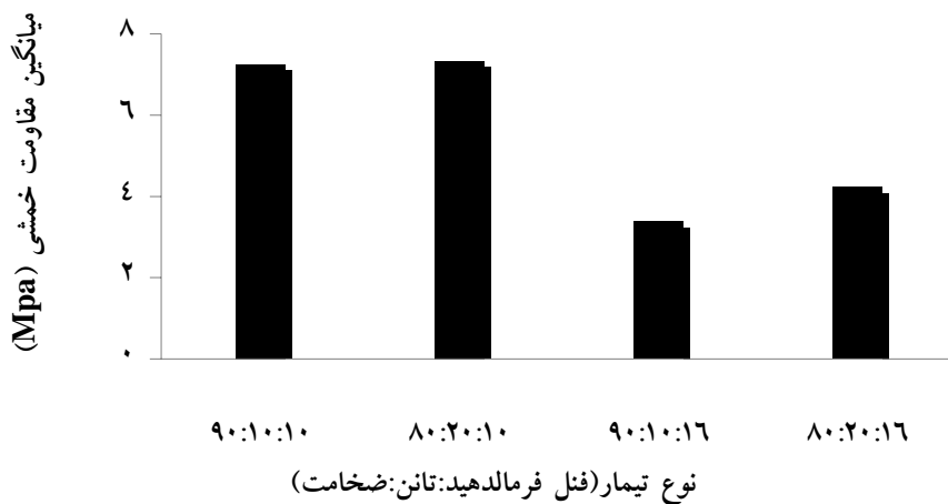
شکل ۱- نمودار میانگین مقاومت خمشی
