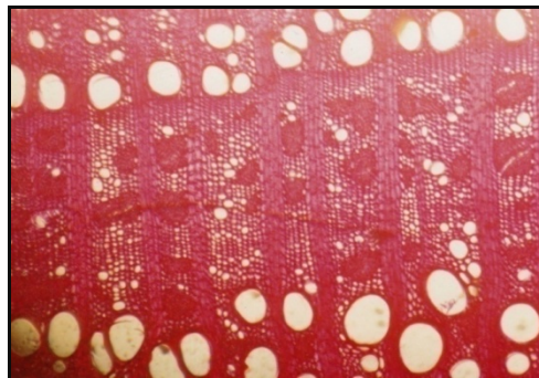
شکل ۸- تصویر میکروسکوپی مقطع عرضی گونه
