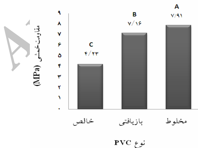
شکل ۱- اثر مستقل نوع PVC بر مقاومت خمشی نمونه‌های آزمایشی
