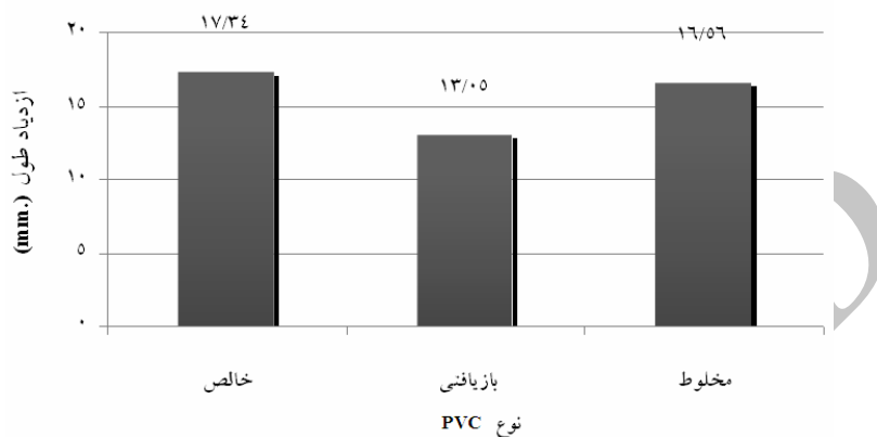
شکل ۴- اثر مستقل نوع PVC بر ازدیاد طول در نقطه تسلیم
