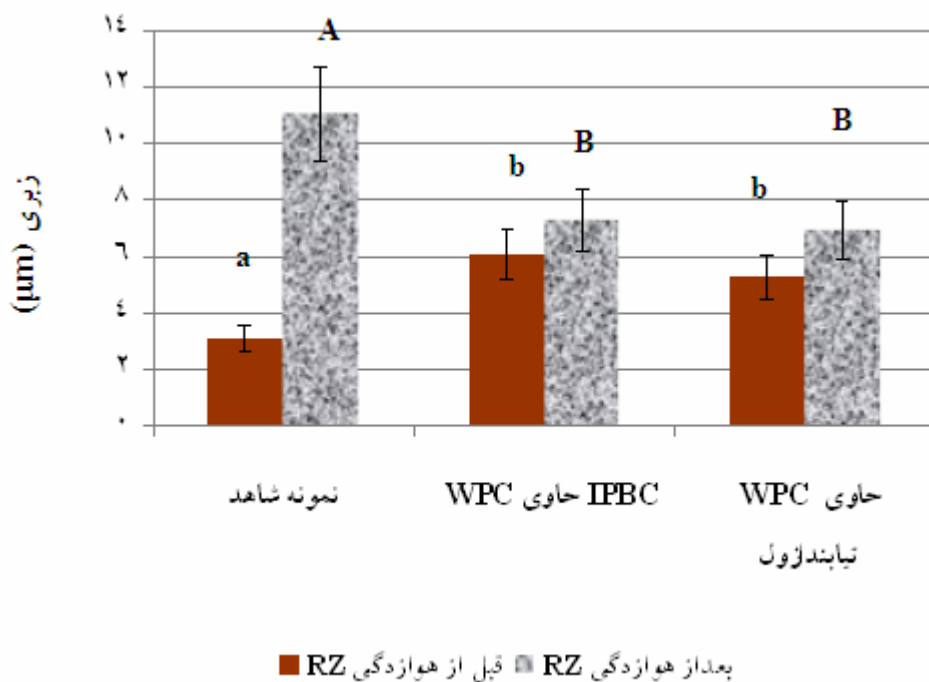
شکل ۳- مقادیر زبری مؤثر (Ra) نمونه شاهد، نمونه حاوی IPBC و نمونه حاوی تیابندزول قبل و بعد از هوازدگی
