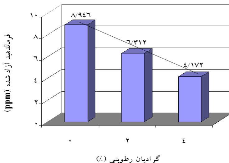
شکل ۲- تأثیر گرادیان رطوبت بر فرمالدهید آزاد شده از تخته خرده چوب زرد تاغ
