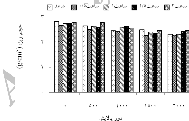
شکل ۳- تغییرات حجم ویژه خمیر کاغذ در سطوح مختلف پالایش و زمان تیمار آنزیمی
