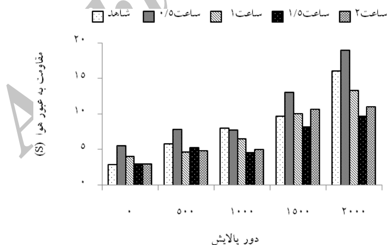
شکل ۶- تغییرات مقاومت به عبور هوای خمیر کاغذ در سطوح مختلف پالایش و زمان تیمار آنزیمی
