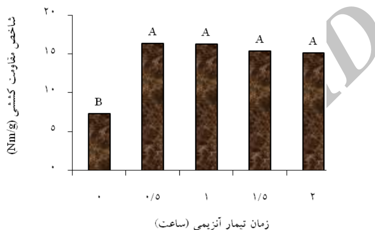
شکل ۸- تغییرات شاخص مقاومت کششی خمیرکاغذ پالایش نشده در زمان‌های مختلف تیمار
