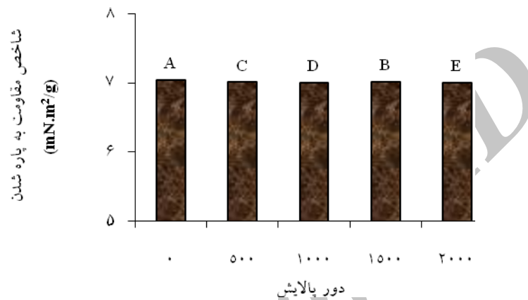
شکل ۱۳- تغییرات شاخص مقاومت به پاره شدن خمیر کاغذ در دوره‌های مختلف پالایش
