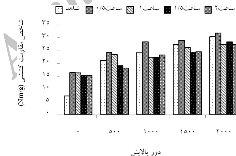
شکل ۹- تغییرات شاخص مقاومت کششی خمیرکاغذ در سطوح مختلف پالایش و زمان تیمار آنزیمی
