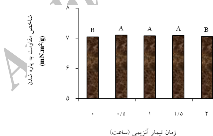
شکل ۱۴- تغییرات شاخص مقاومت به پاره شدن خمیر کاغذ پالایش نشده در زمان‌های مختلف تیمار
