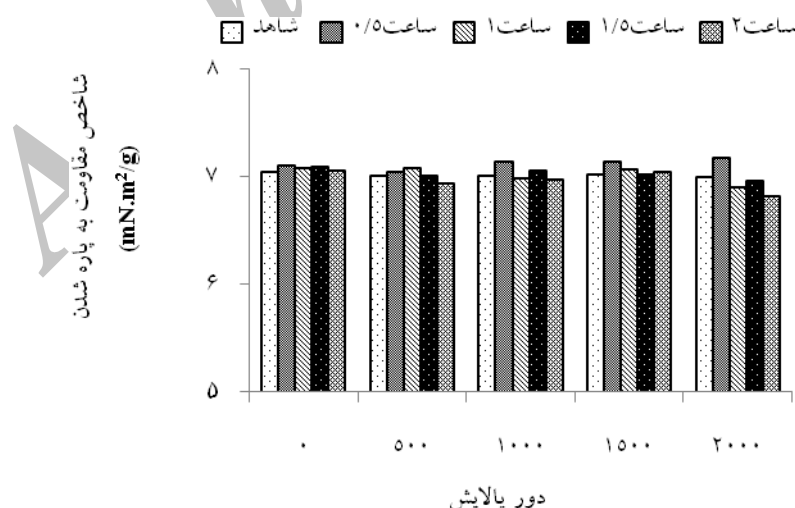
شکل ۱۵- تغییرات شاخص مقاومت به پاره شدن خمیرکاغذ در سطوح مختلف پالایش و زمان تیمار آنزیمی
