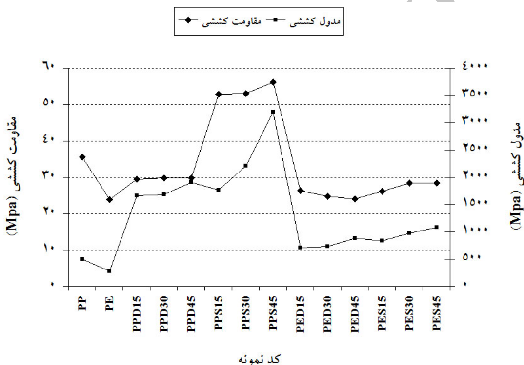
شکل ۱- تأثیر نوع پلیمر، پرکننده و میزان پرکننده بر مقاومت و مدول خمشی چندسازه ویژگی‌های کششی (مقاومت و مدول)
