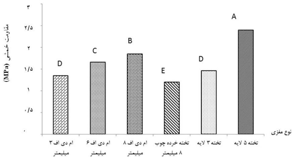
شکل ۲- اثر مستقل نوع پوسته بر مقاومت خمشی
