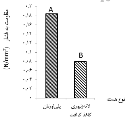
شکل ۹- اثر مستقل نوع مغزی بر مقاومت به فشار
