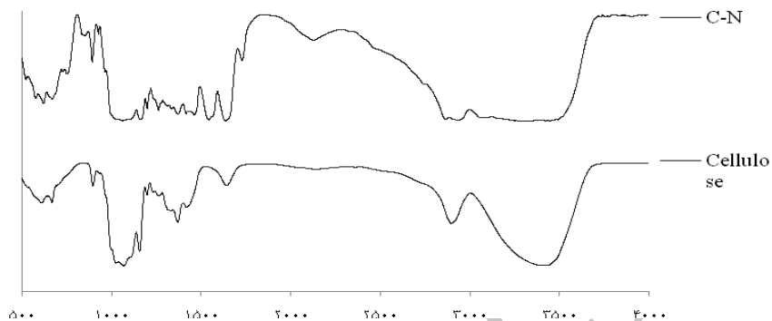
شکل ۷- طیف مادون قرمز چندسازه‌های سلولزی؛ C: سلولز و C-N: سلولز-نایلون
