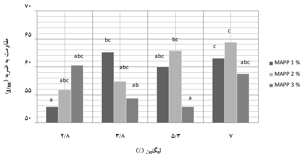
شکل 5- تغییر مقاومت به ضربه چندسازه الیاف سلولزی پلی پروپیلن در اثر تغییر مقدار لیگنین و MAPP
