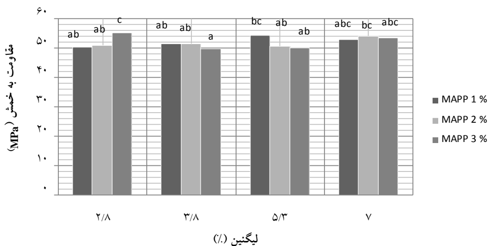
شکل 3 تغییر مقاومت خمشی چندسازه الیاف سلولزی پلی پروپیلن در اثر تغییر مقدار لیگنین و MAPP
