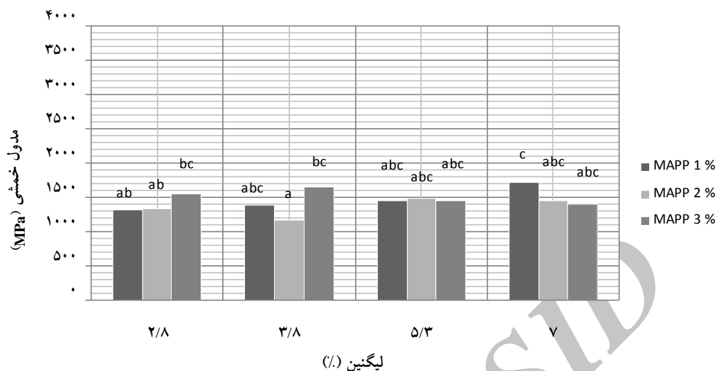
شکل 4 تغییر مدول الاستیسیته خمشی چندسازه الیاف سلولزی پلی پروپیلن
