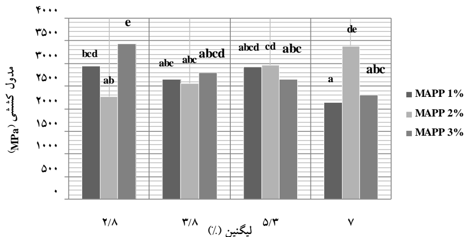
شکل 2 تغییر مدول الاستیسیته کششی چندسازه الیاف سلولزی پلی پروپیلن در اثر تغییر مقدار لیگنین و MAPP و گروه بندی دانکن میانگین های مقاومت خمشی در شکل 3 تأثیر متقابل عوامل مورد بررسی بر ویژگی های خمشی چندسازه نیز در سطح اعتماد آماری 99 درصد معنی دار شده و مدول الاستیسیته خمشی در شکل 4 آورده شده است.
