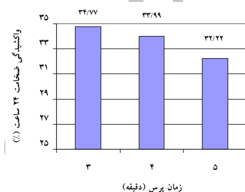
شکل 5 اثر مستقل زمان پرس بر واکسیدگی ضخامت 2 و 24 ساعت
