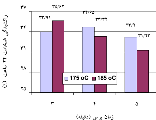
شکل 6 اثر متقابل دما و زمان پرس بر واکسیدگی ضخامت 2 و 24 ساعت
