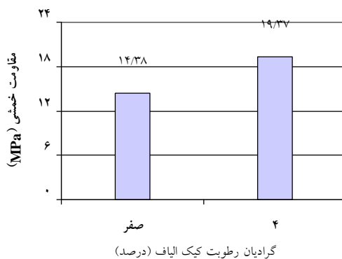
شکل 1 تأثیر گرادیان رطوبت کیک الیاف بر مقاومت خمشی
