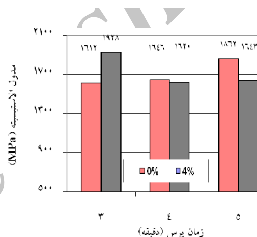
شکل 2 اثر متقابل گرادیان کیک الیاف و زمان پرس بر مقاومت خمشی و مدول الاستیسیته
