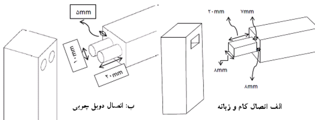
شکل 2- ابعاد و طرح اتصال: الف کام و زبانه و ب دوبل چوبی
