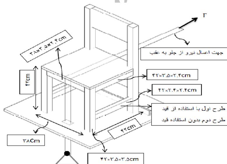
شکل 1 - طرح و ابعاد صندلی آزمونی به همراه روش اعمال نیرو از جلو به عقب
