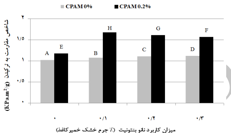
شکل ۲- تأثیر سامانه نانوبنتونیت/نشاسته کاتیونی/CPAM بر شاخص ترکیدن کاغذ
