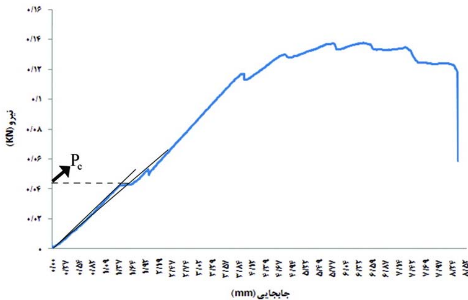
شکل ۷- طرح شماتیکی از ارتباط نیرو و تغییر مکان تحت آزمون مکانیک شکست (در هر دو منحنی خط سمت چپ نشان دهنده شیب آغازین در ناحیه الاستیک و خط دوم، خطی با شیب ۹۵٪ شیب آغازین است)
