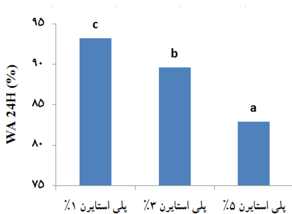
شکل ۵- اثر درصد پلی‌استایرن بر روی جذب آب بعد از ۲۴ ساعت غوطه‌وری در آب
