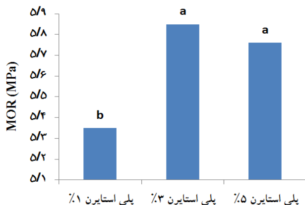
شکل ۲- تأثیر مقدار پلی‌استایرن بر روی مقاومت خمشی
