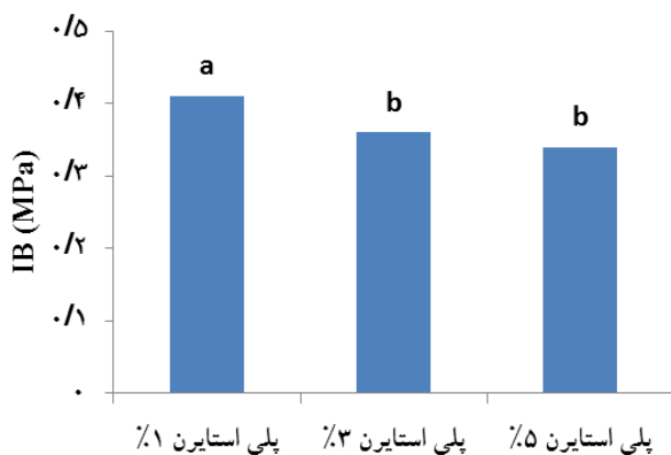
شکل ۱- اثر درصد پلی‌استایرن بر روی چسبندگی داخلی
