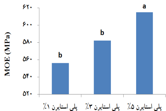
شکل ۳- اثر درصد پلی‌استایرن بر روی مدول الاستیسیته
