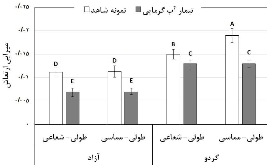
شکل ۳- میرایی ارتعاش گونه‌های آزاد و گردوی تیمار آب گرمایی شده تحت ارتعاش در جهت‌های طولی - شعاعی و طولی - مماسی
