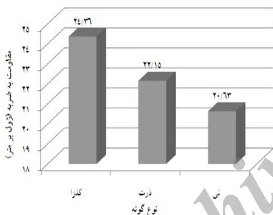
شکل ۷- اثر مستقل ماده سلولزی بر مقاومت به ضربه چندسازه چوب
