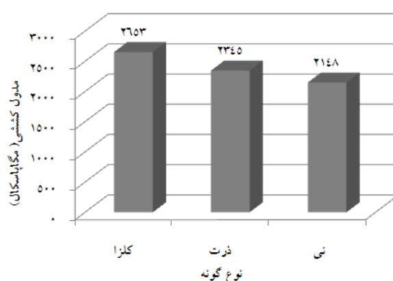
شکل ۱- اثر مستقل نوع ماده سلولزی بر خواص کششی چندسازه چوب پلاستیک
