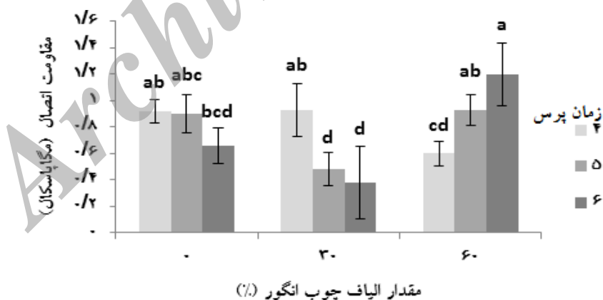
شکل ۷- اثر متقابل درصد اختلاط الیاف چوب انگور و زمان پرس بر مقاومت اتصال روکش به سطح نمونه
