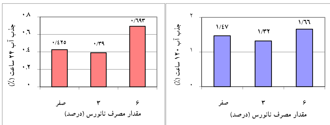
شکل ۸- اثر مستقل مصرف نانورس بر جذب آب ۲۴ و ۱۲۰ ساعت
