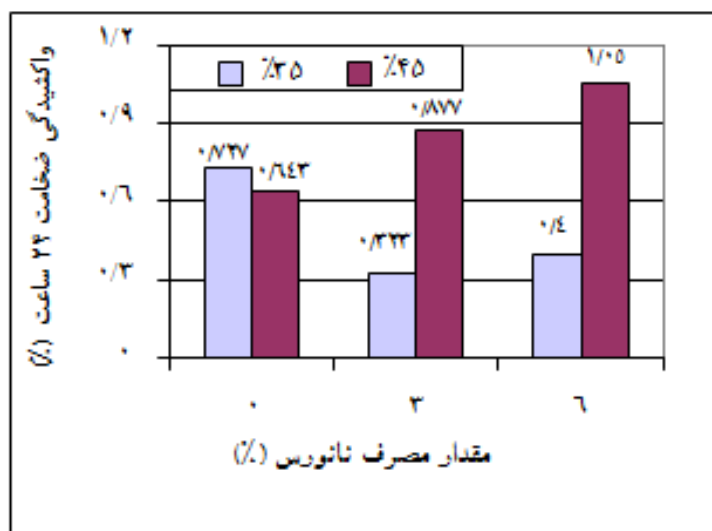
شکل ۷- اثر متقابل مقدار مصرف آرد ساقه سویا و نانورس بر واکسیدگی ضخامت ۲۴ ساعت
