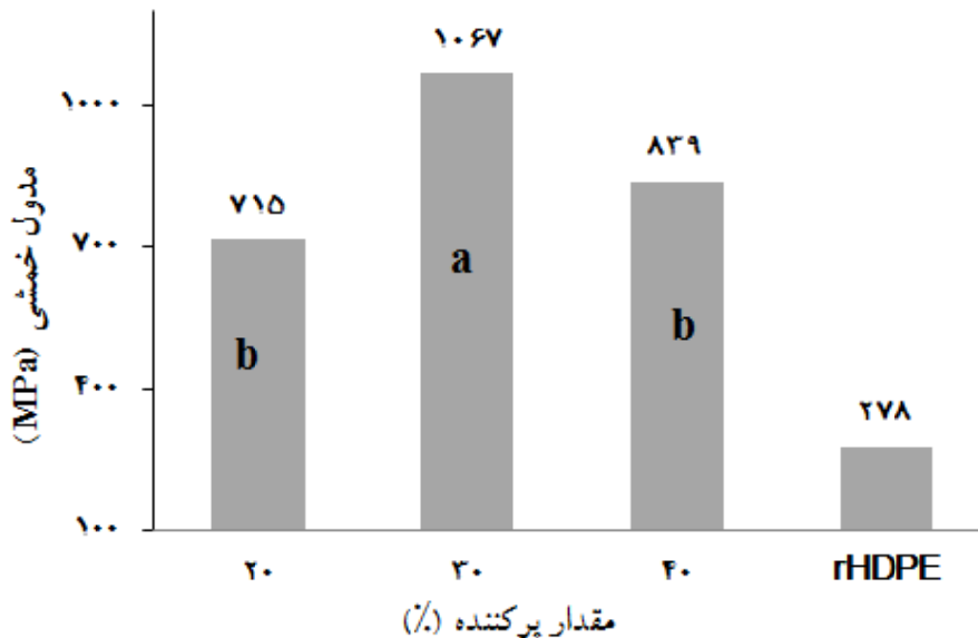
شکل ۴- تأثیر مقدار پرکننده بر مدول خمشی
