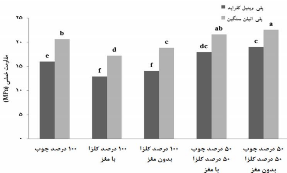
شکل ۳- اثر متقابل نوع پلیمر و نوع ماده لیگنوسلولزی بر مقاومت خمشی چندسازه چوب پلاستیک
