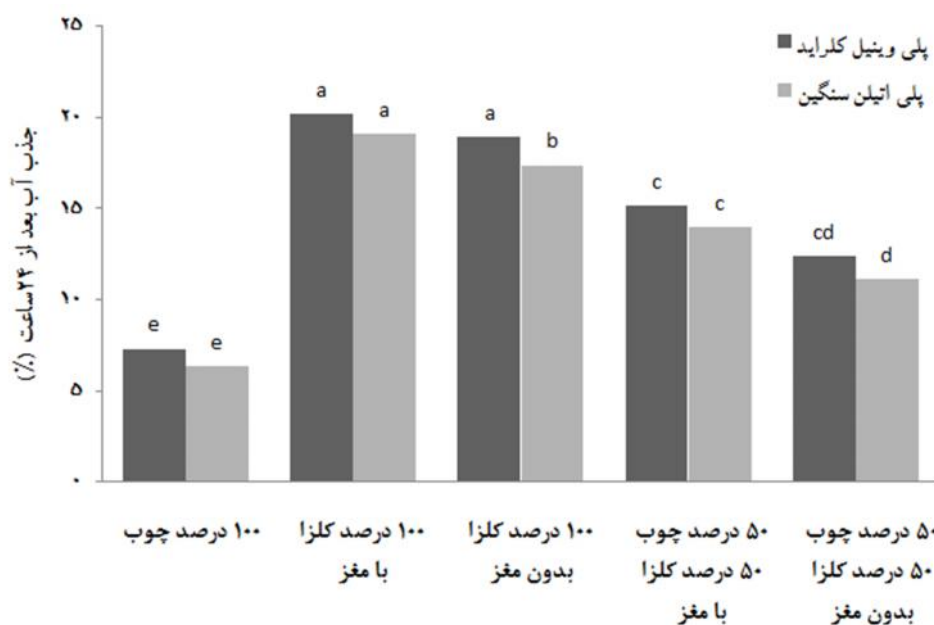
شکل ۲- اثر متقابل نوع پلیمر و نوع کیفیت ماده لیگنوسولوزی بر جذب آب ۲۴ ساعت
